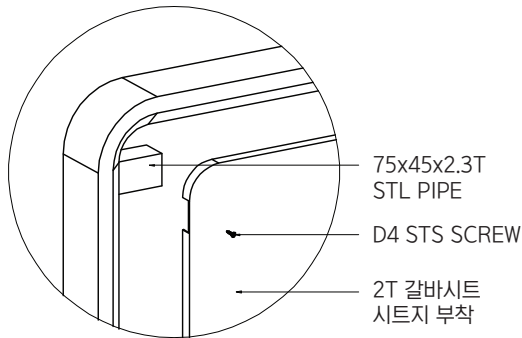
5 DETAIL A-A 088 SCALE : NONE
