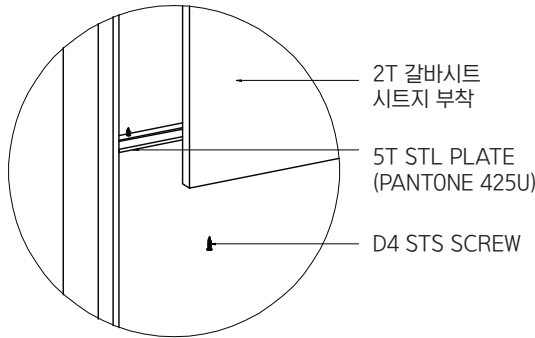
6 DETAIL A-B 088 SCALE : NONE
