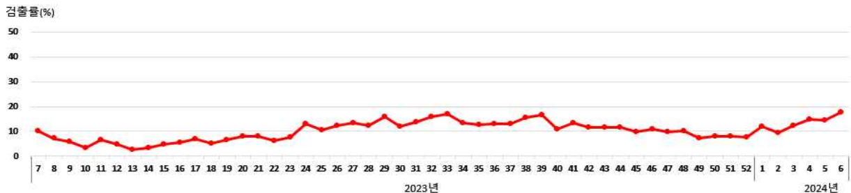
< 코로나19 검출현황 ('23.12.~'24.2.10.) >
